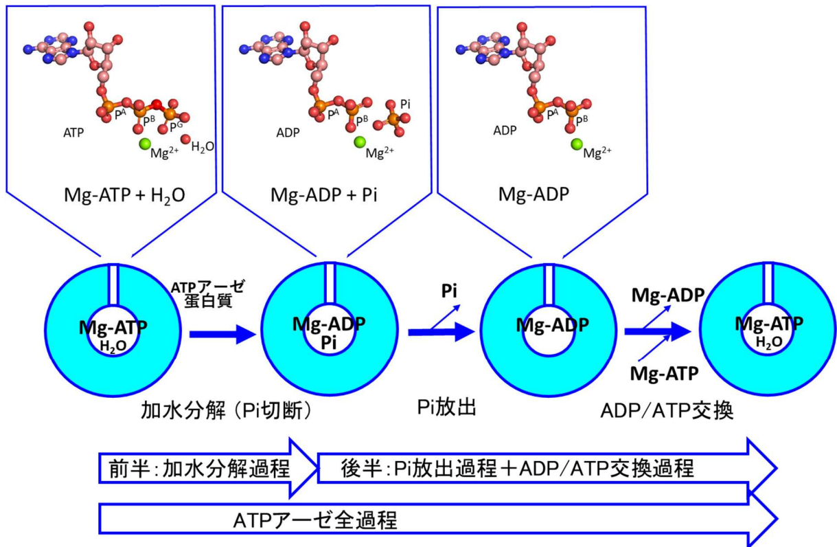
図 3. ATP アーゼ蛋白質は ATP アーゼ過程によって蛋白質分子内に結合した ATP を加水分解し(前半過程)、さらに分解産物(PiとADP)を放出する(後半過程)。上段は、Mg-ATP, Mg-ADP-Pi, Mg-ADP の構造:炭素(桃色)、窒素(青)、リン(朱)、酸素(赤)の各原子と Mg 2+ (緑)。
